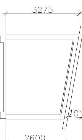
SEKTION GÄSTSTUGA
