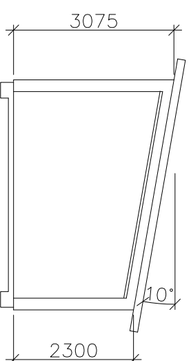
SEKTION ATTEFALLSHUS
